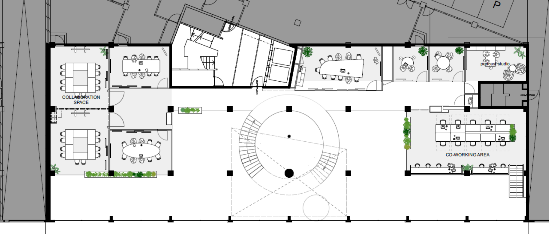
1 ENTRESOL_GEBOUW B_LAYOUT
